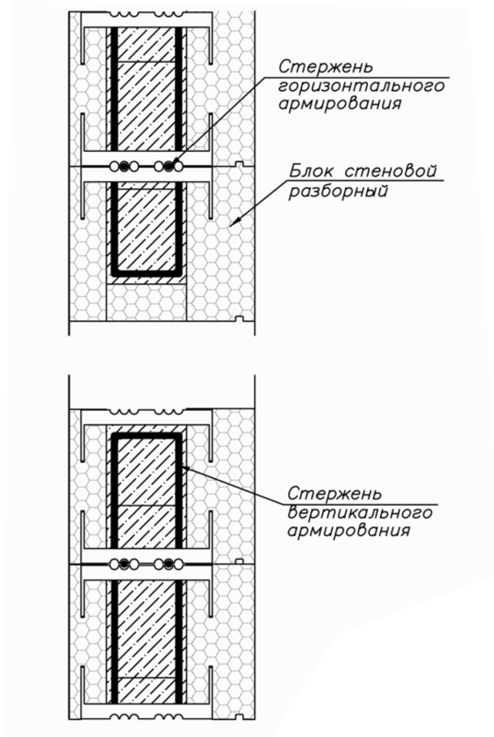
Узел армирования стен в зоне проема
