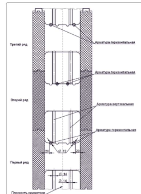
Рис.6 Армирование стен
