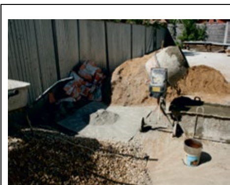
Рис.9 Приготовление бетона на строительной площадке
