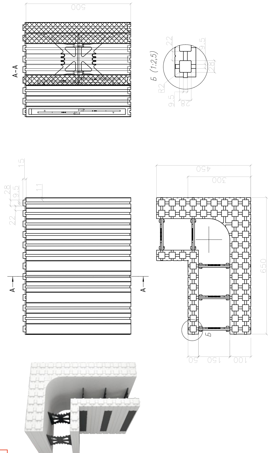
Блок стеновой угловой (левый) 50 серия
