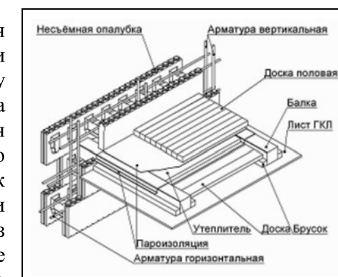
Рис.11 Деревянное перекрытие
