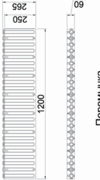
Элемент блока разборного - 110
