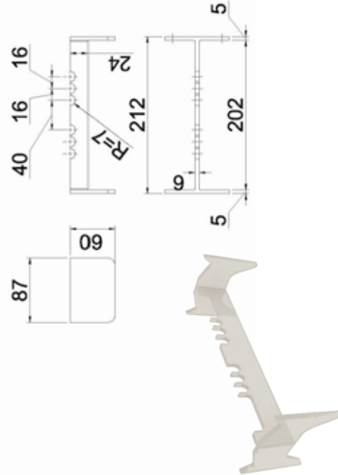
Перемычка для блоков разборных
