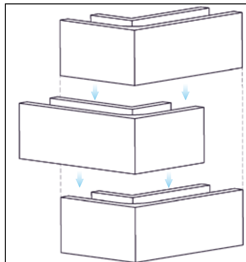
Рис.4 Монтаж угловых блоков несъемной опалубки
