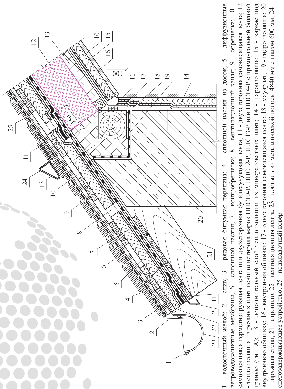
Рисунок А.11.3 - Карниз крыши (Узел 2)
