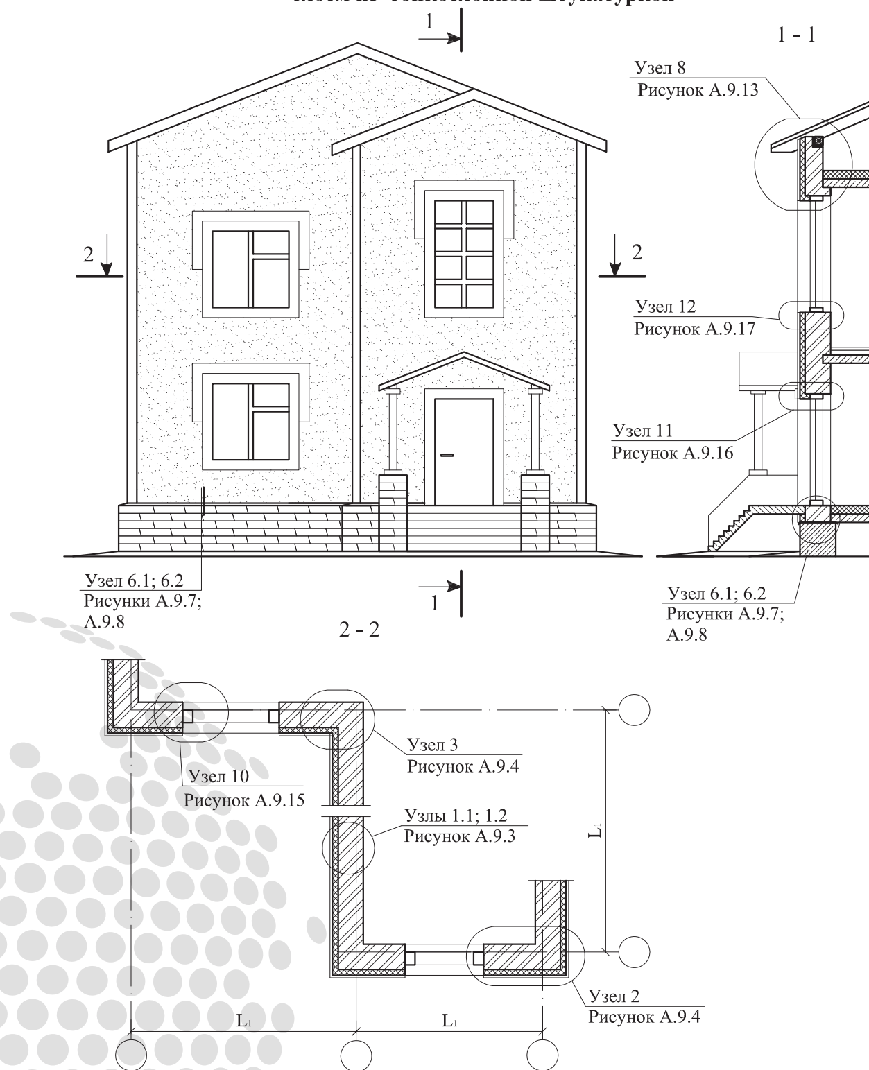
Рисунок А.9.1 - Фасад здания, разрезы 1-1 и 2-2
