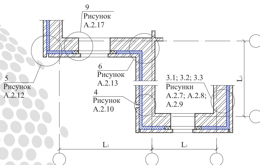
Рисунок А.2.2 - Схема расположения плит теплоизоляции и противопожарных рассечек
