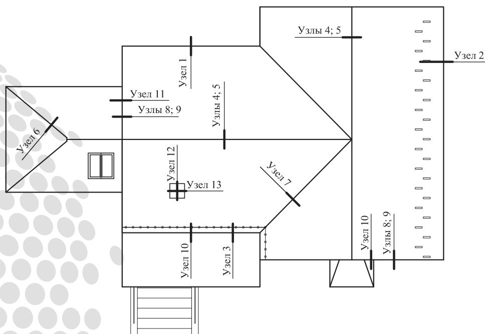
Рисунок А.11.1 - План крыши коттеджа и нумерация узлов
